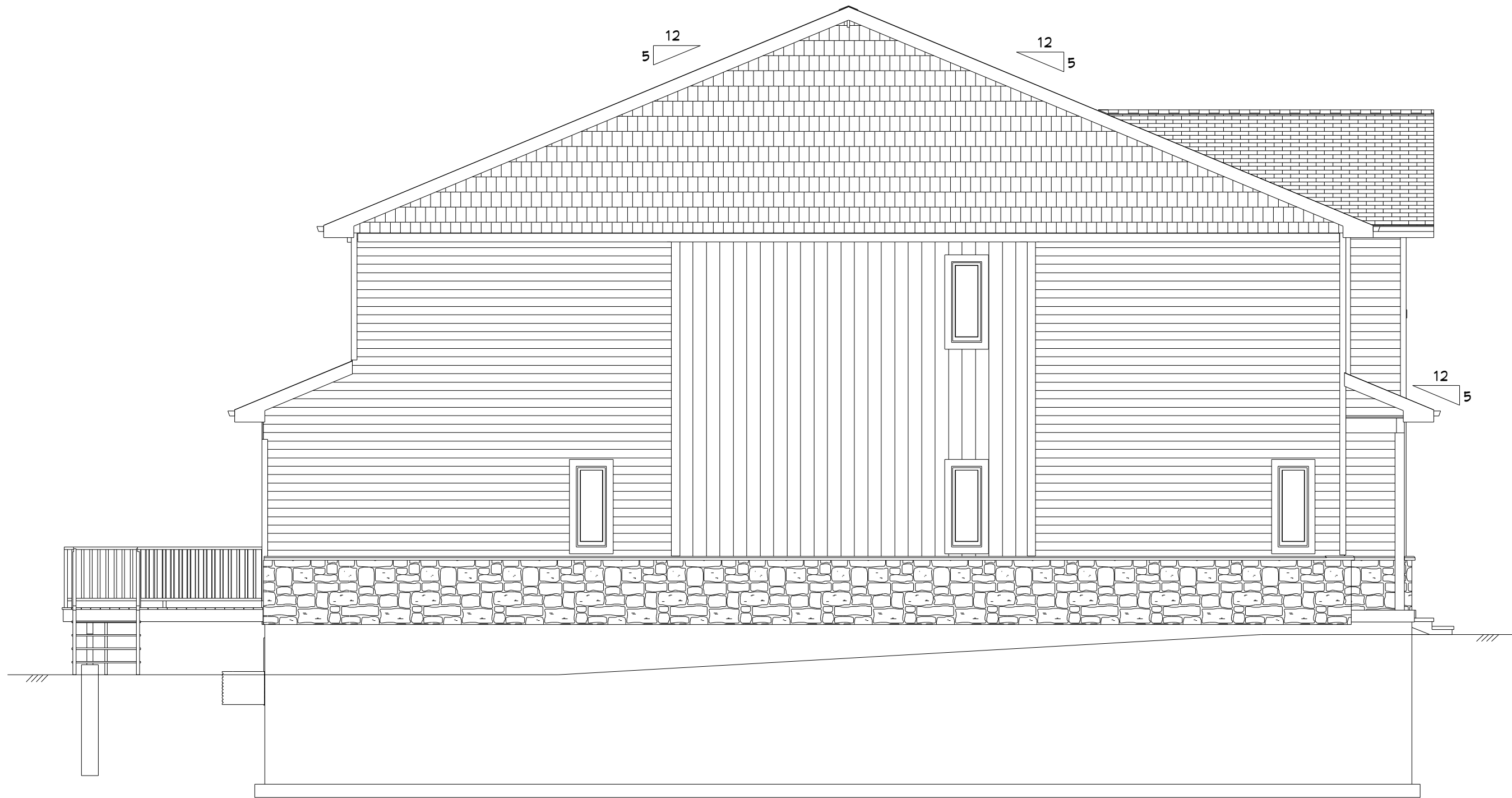
(E3) Elevation - Right
