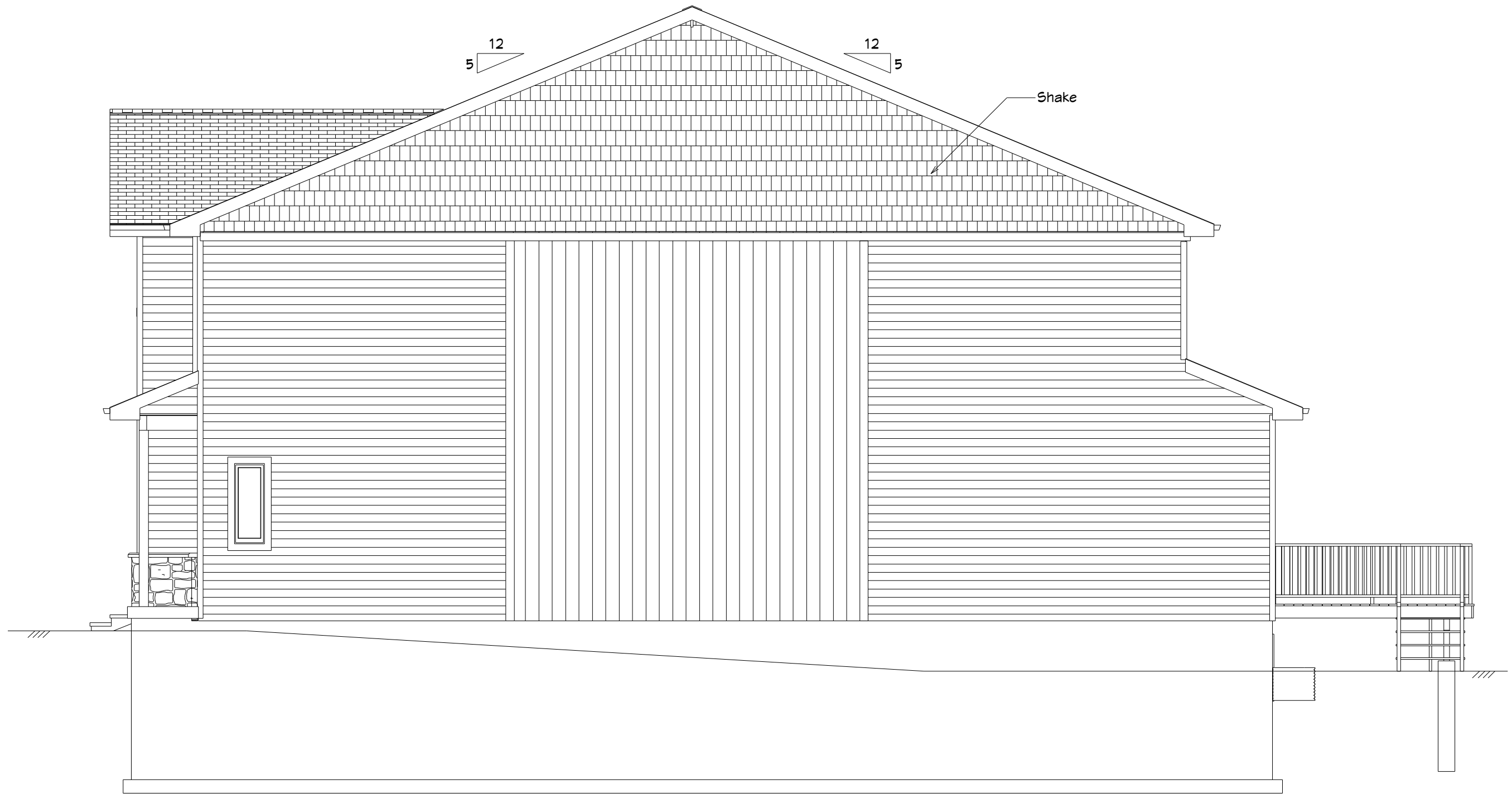
ⓔ2 Elevation - Right
